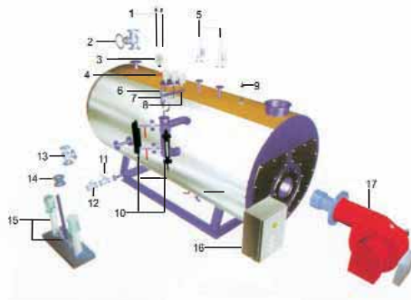
Nyomás legfeljebb 18 bar
