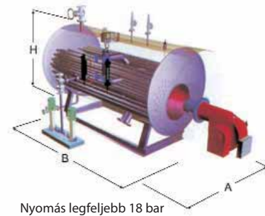
Nyomás legfeljebb 18 bar
